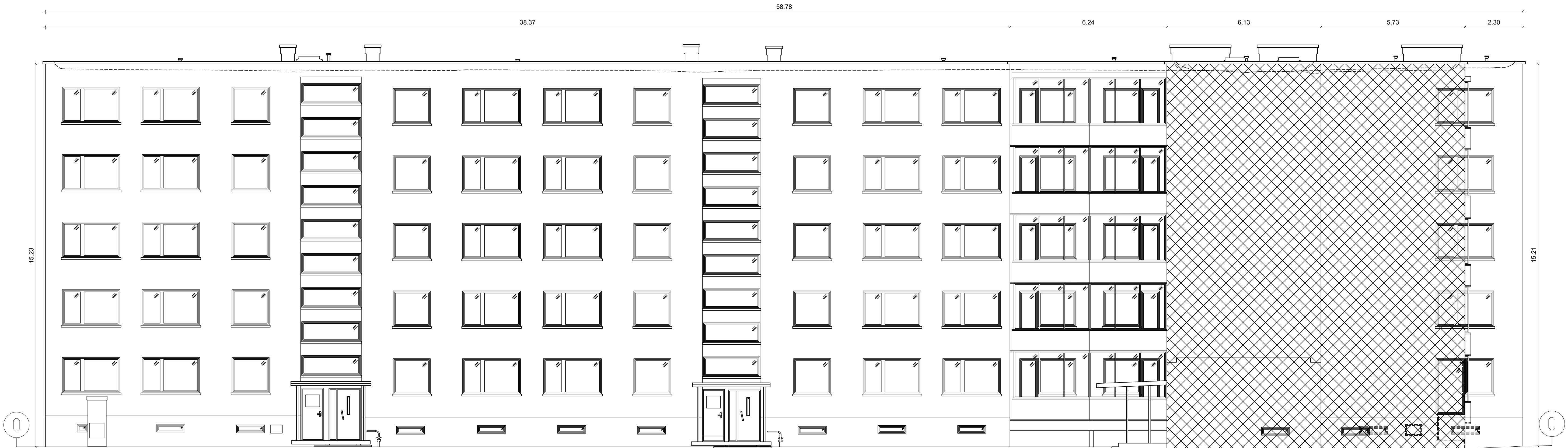
A FASADAS 1:100
